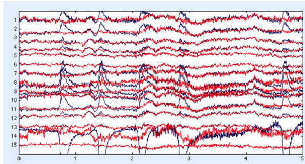
EEG
